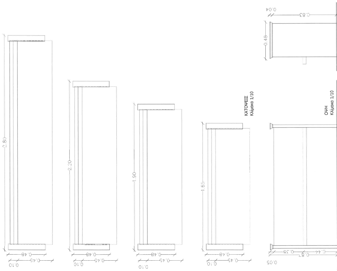
ΠΑΛΙΑ ΟΥΨΗ Κλίμακα 1/10
