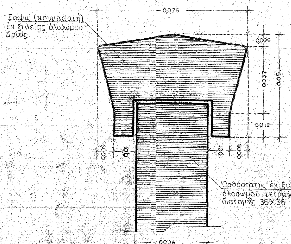
ΒΗΜΑ ΜΑΡΤΥΡΟΣ ΜΕΤΑ ΒΑΘΡΟΥ ΤΟΜΗ Β-Β κλ. 1/10
