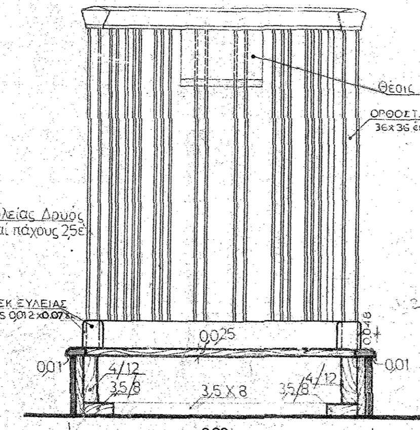
ΒΗΜΑ ΜΑΡΤΥΡΟΣ ΜΕΤΑ ΒΑΘΡΟΥ ΤΟΜΗ Β-Β κλ. 1/10
