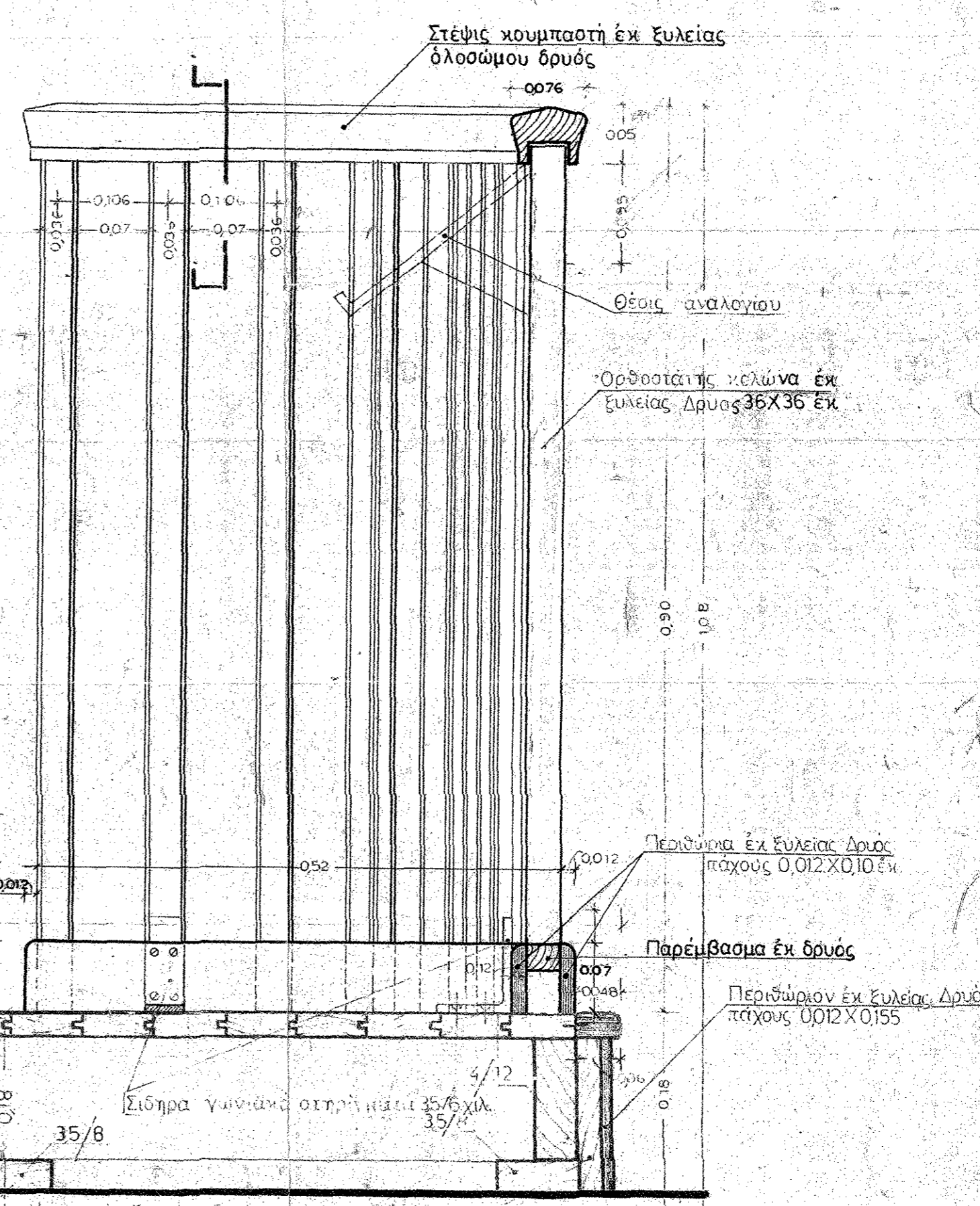
ΒΗΜΑ ΜΑΡΤΥΡΟΣ ΜΕΤΑ ΒΑΘΡΟΥ ΤΟΜΗ Α-Α κλίμαξ 1/5
