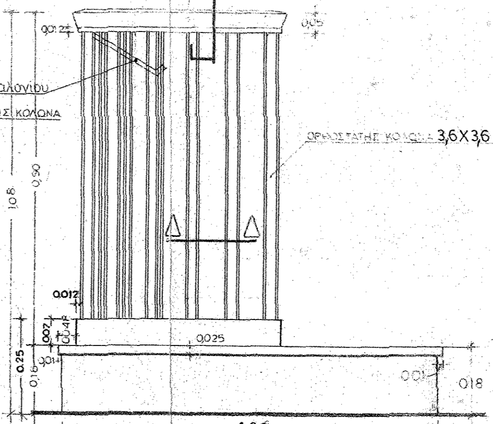
ΒΗΜΑ ΜΑΡΤΥΡΟΣ ΜΕΤΑ ΒΑΘΡΟΥ ΠΛΑΓΙΑ ΟΨΙΣ κλ. 1/10
