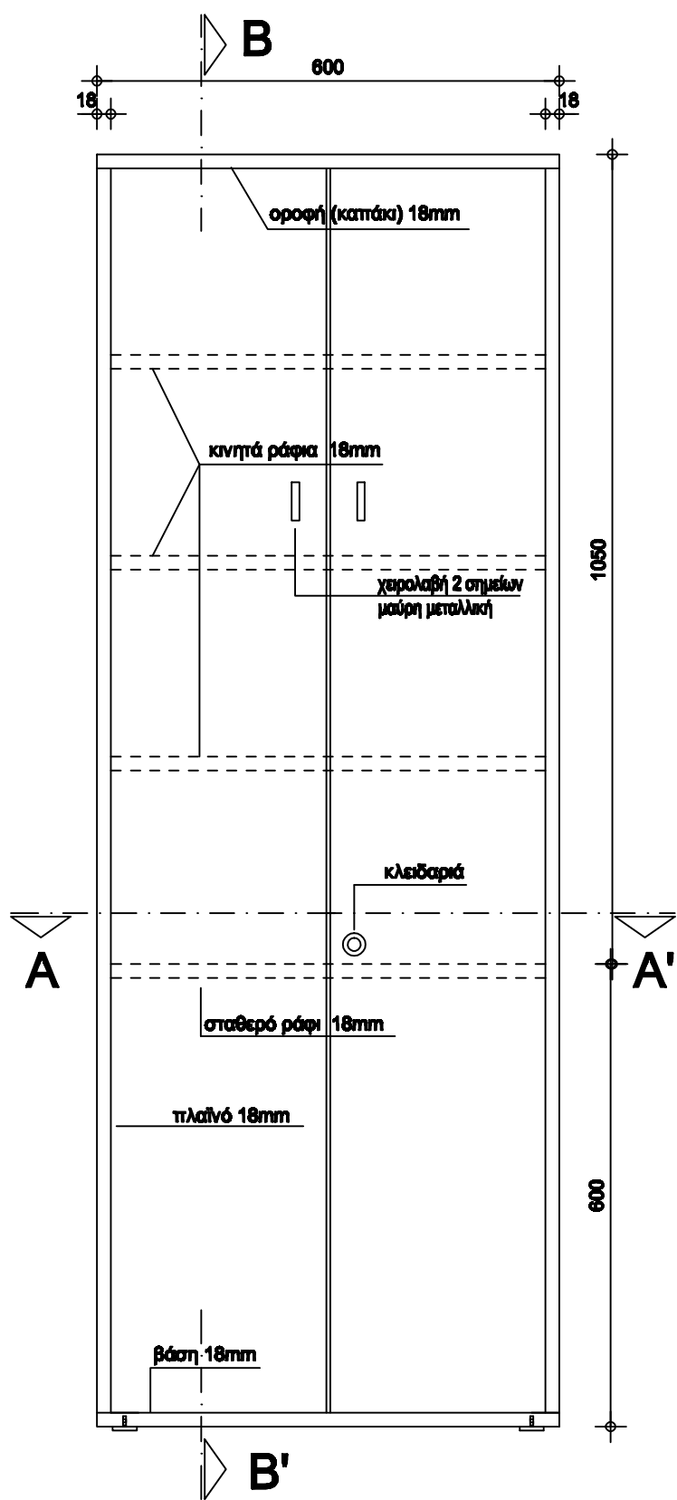
ΟΨΗ ΒΙΒΛΙΟΘΗΚΗΣ
