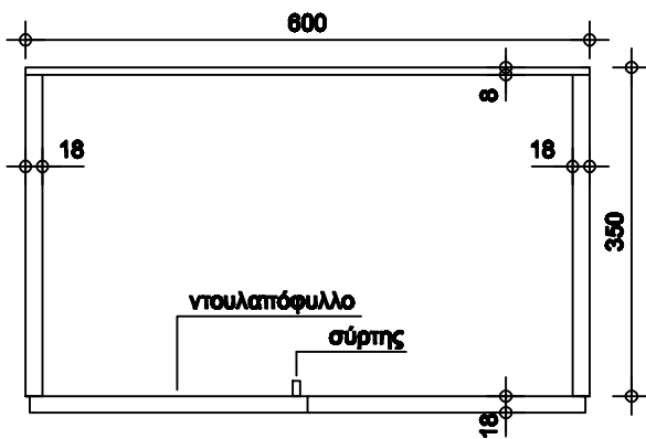
ΤΟΜΗ Α-Α'
