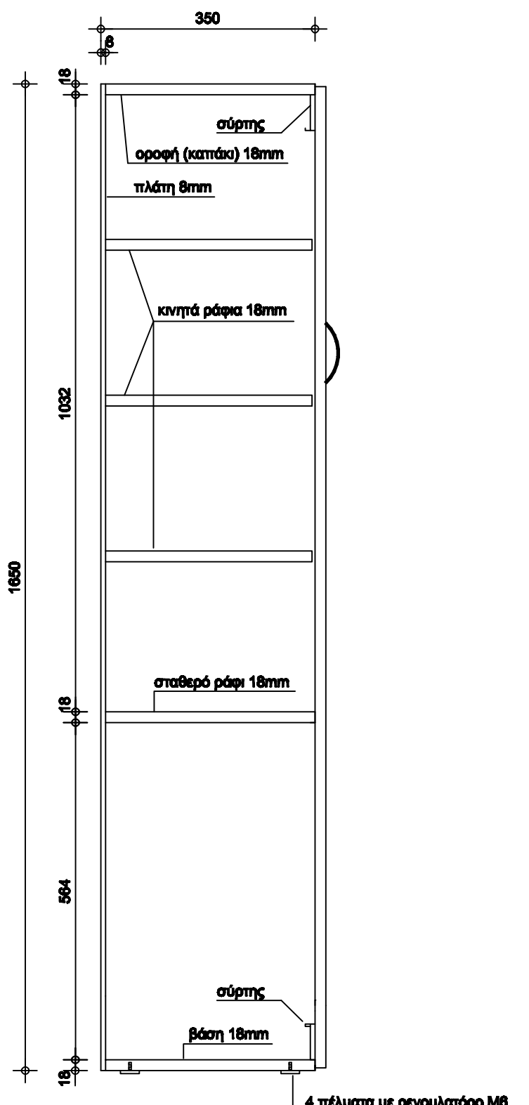
ΤΟΜΗ Β-Β'
