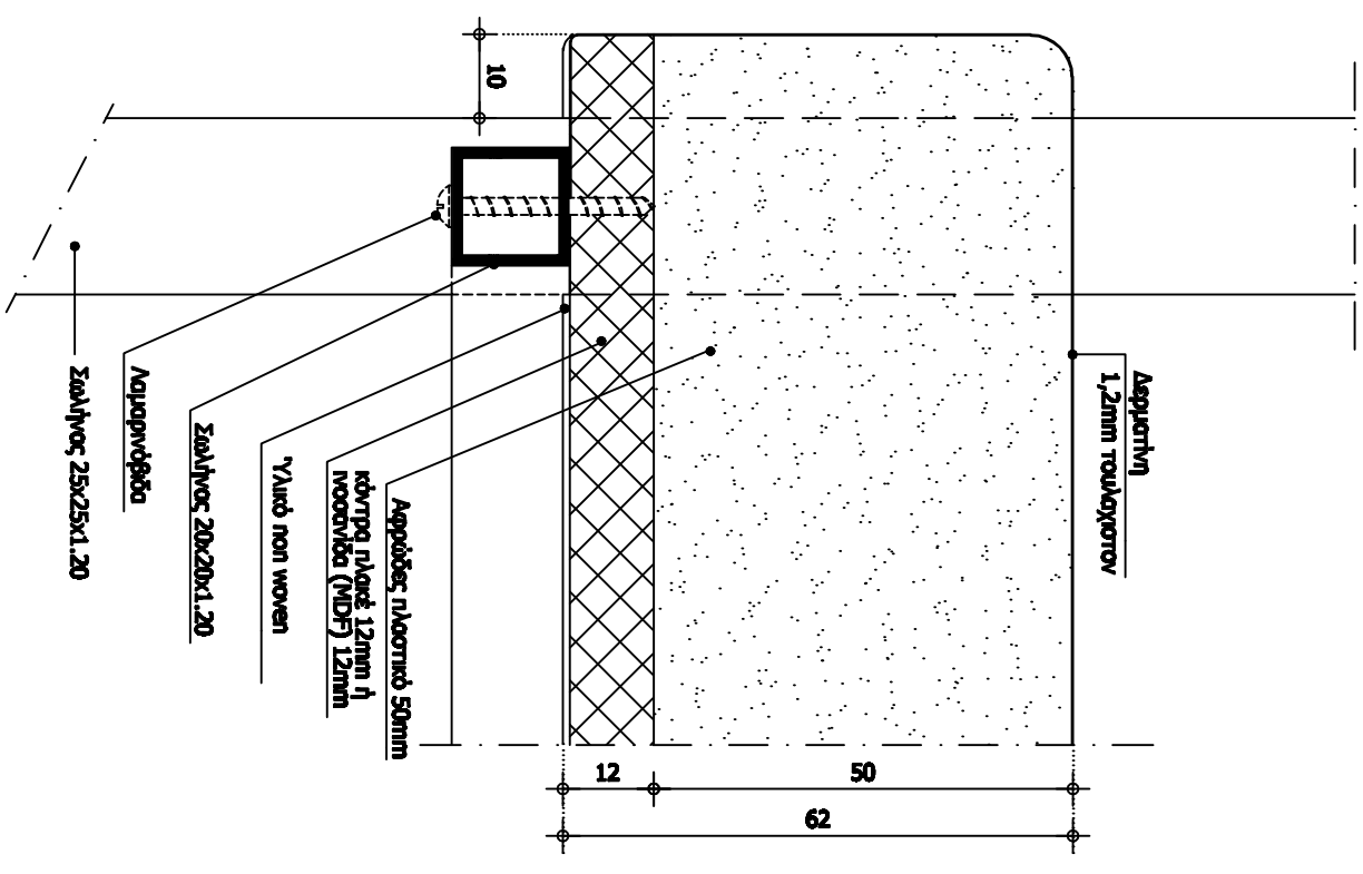
ΑΕΤΤΟΜΕΡΕΙΑ Γ' (Τομή στην έδρα του καθίσματος) ΚΛΙΜΑΚΑ 1:1
