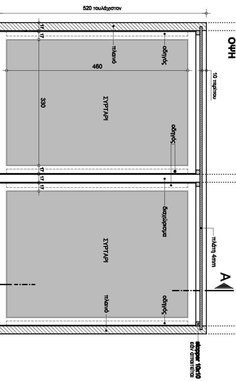
ΟΡΙΖΟΝΤΙΑ ΤΟΜΗ Β-Β (εναλλακτική πρόταση 2 ή 1α)
